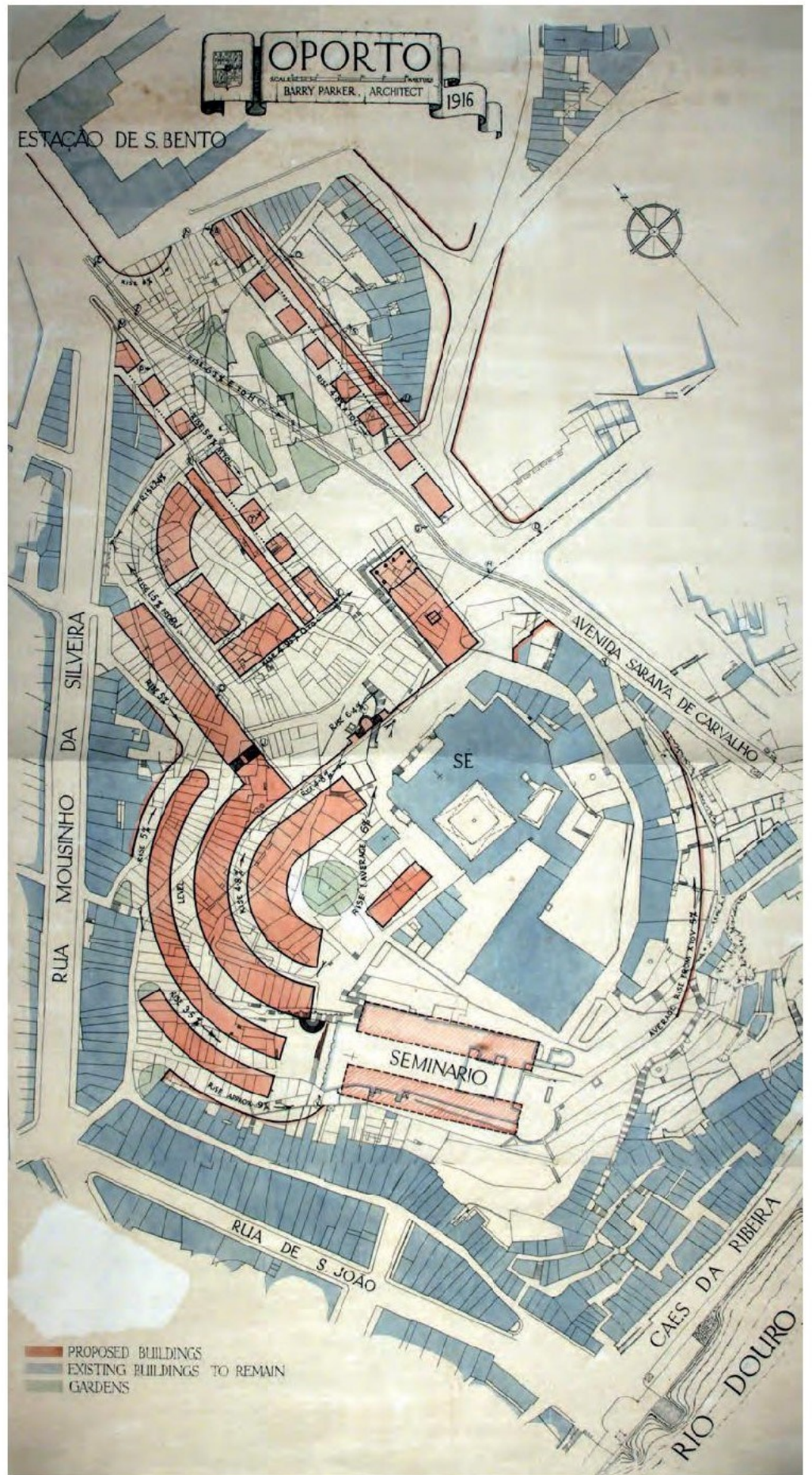
Plano de Barry Parker para a Avenida da Ponte (1916)
